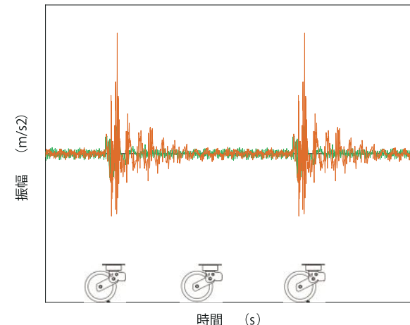
時間軸波形
